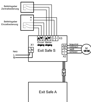
Abbildung 1: Schematischer Anschlussplan
