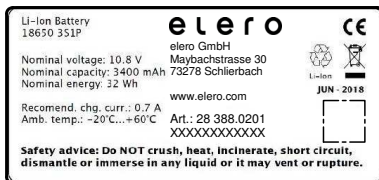
Abbildung 3: Typenschild Akkupack
