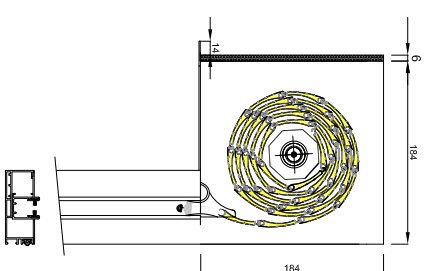
Kastengröße 180 mit Insektenschutz bis Rollladenhöhe 2350mm ohne Insektenschutz bis Rollladenhöhe 2850mm
