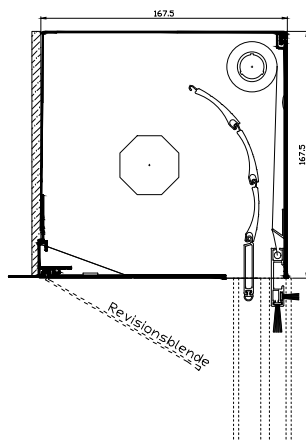
Kastengröße 165 mit I-Rollo
