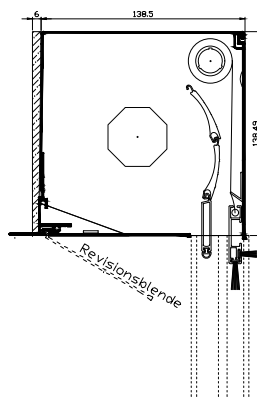
Kastengröße 138 mit I-Rollo
