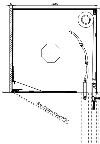
Kastengröße 180 mit I-Rollo
