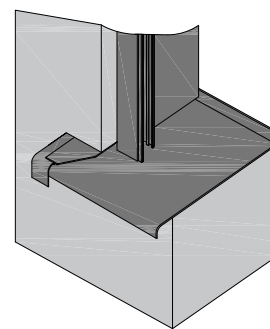
newoPro Führungsschiene Typ B Teilverputz
