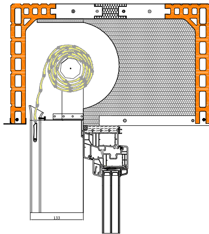
newoPro Führungsschiene Typ A
