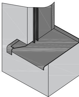
newoPro Führungsschiene Typ A Unterputz
