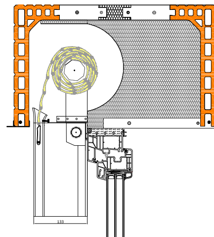
newoPro Führungsschiene Typ A mit Insektenrollo
